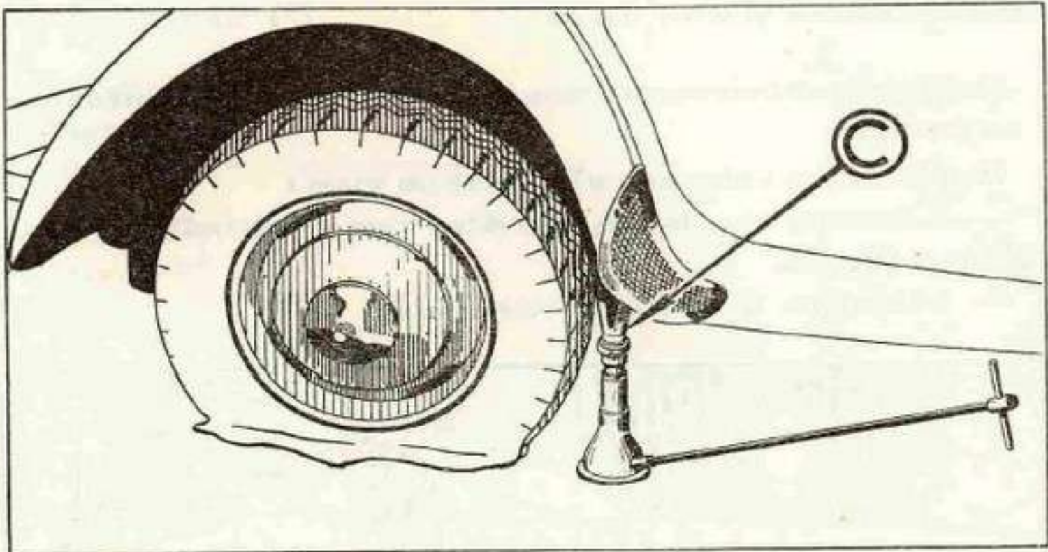
Fig. 6. — POSITION DU CRIC A L'ARRIÈRE.
