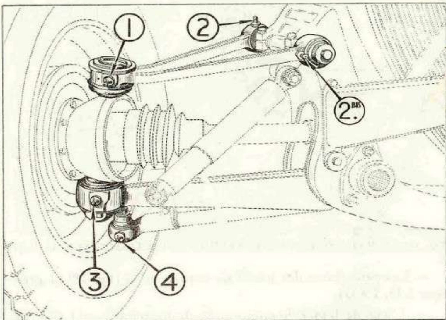
Fig. 12. — GRAISSEURS DU TRAIN AV.
