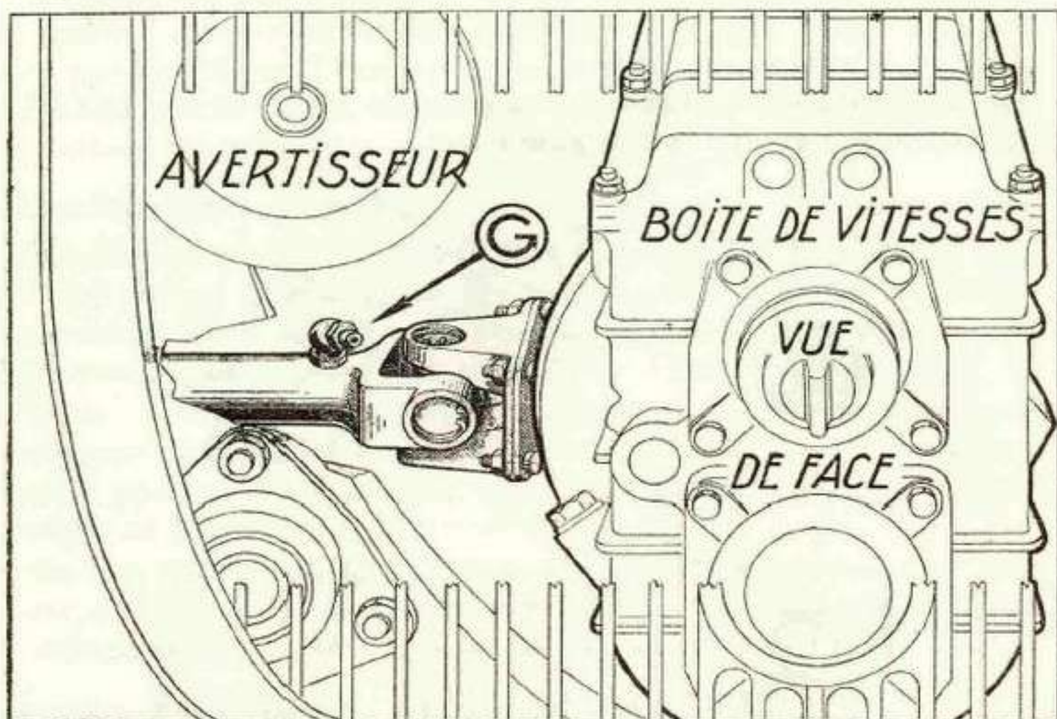
Fig. 13. — GRAISSEUR DES CANNELURES DE CARDAN SUR 11 B (1).
