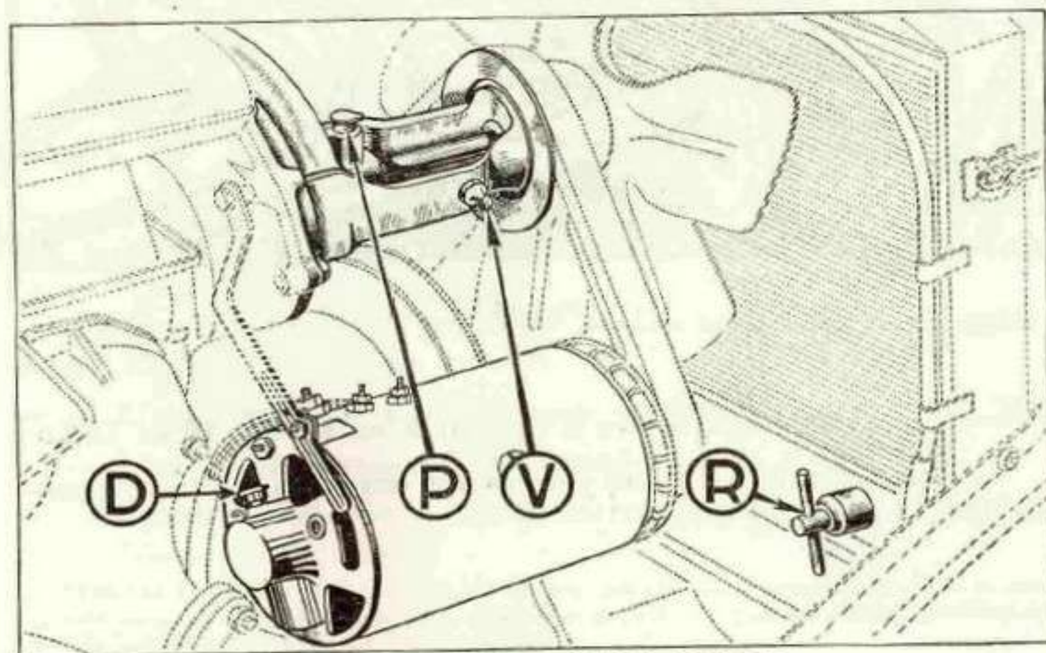
Fig. 16. — DYNAMO PARIS-RHONE
