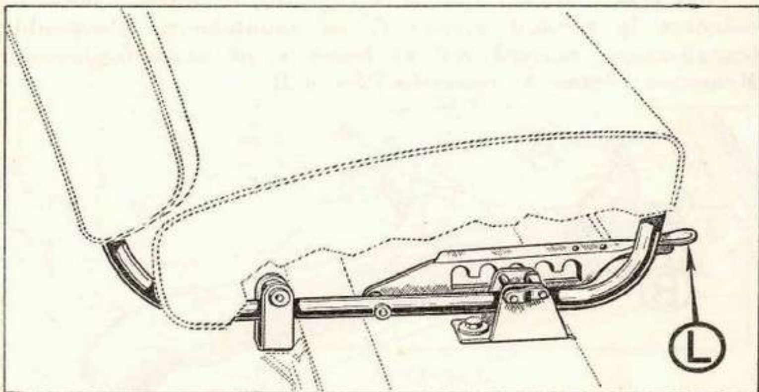
Fig. 9. — RÉGLAGE DES SIÈGES AVANT.
