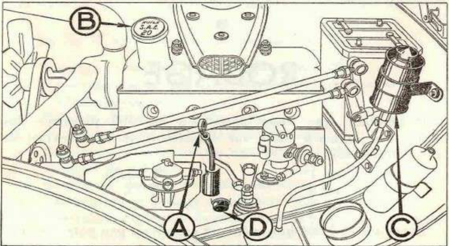
Fig. 1. — JAUGE D'HUILE (A). — ORIFICE DE REMPLISSAGE (B). RÉSERVOIR DU LIQUIDE POUR FREINS (C).
