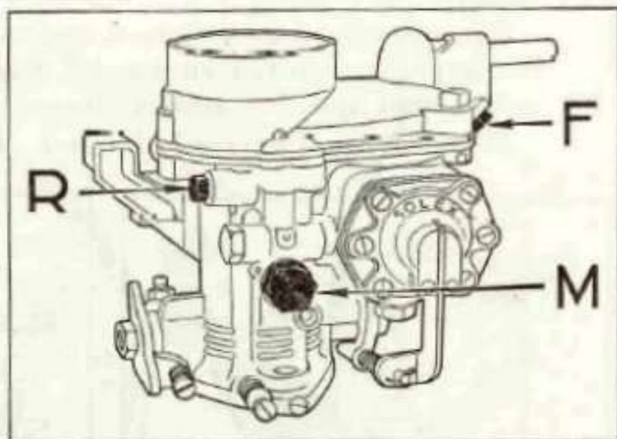
CARBURATEUR SOLEX 33 PBIC
